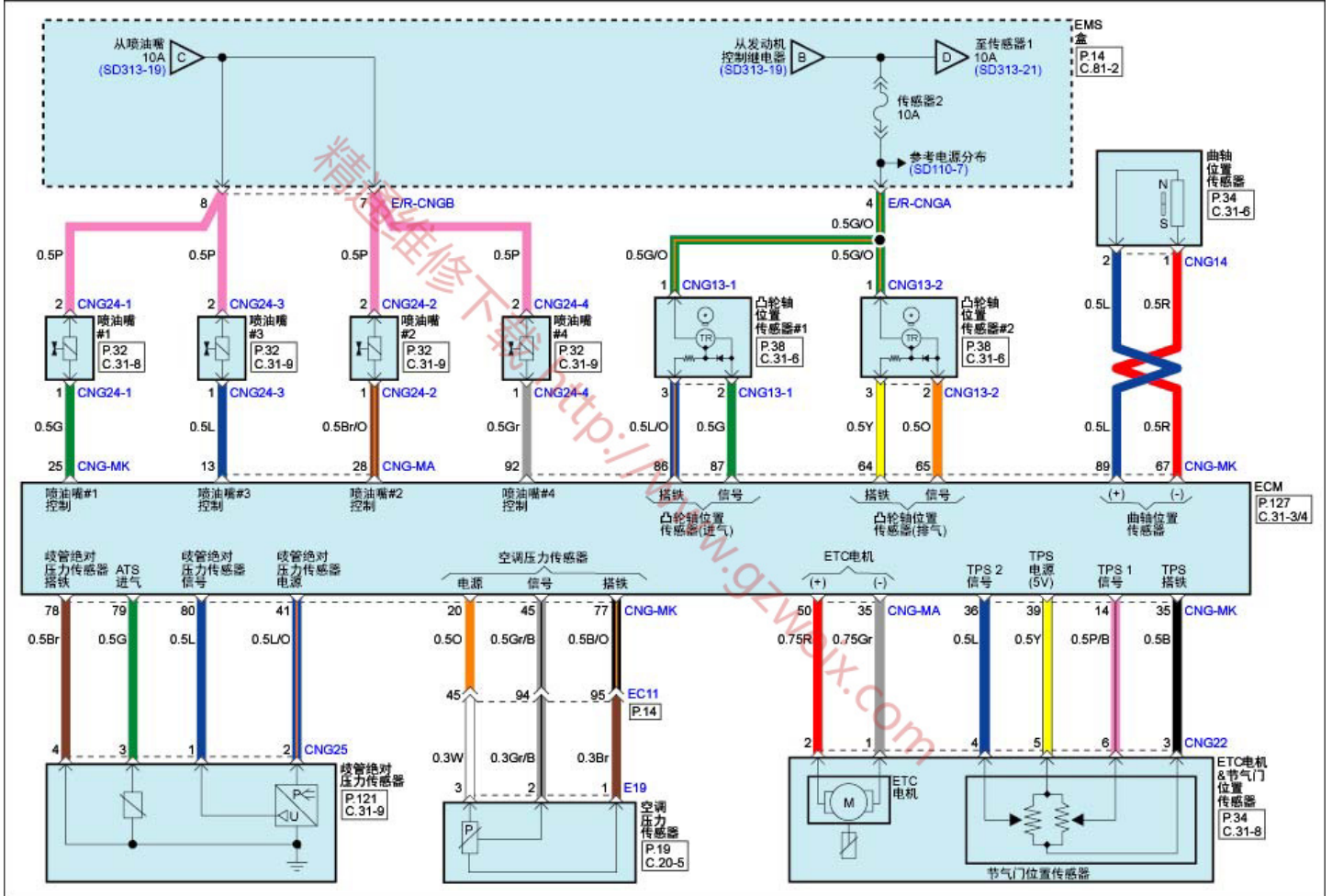
发动机控制系统(G4NB : NU 1.8L MPI M/T)(4)
